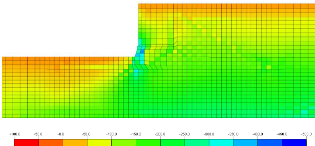
a) 最小主応力図
