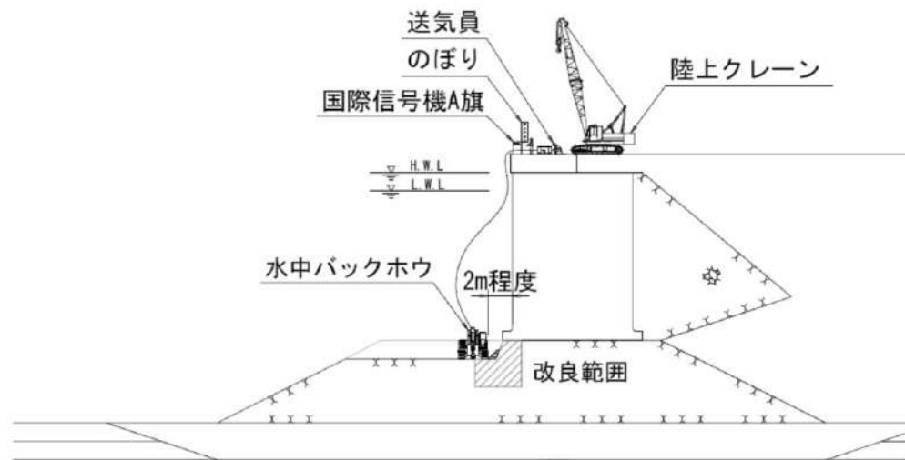
図-5.5.3 水中バックホウによる係船岸付近の捨石撤去状況
