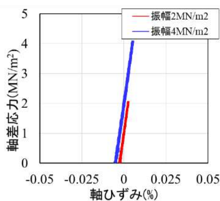
b) Case1 : 地震荷重(2,4 MN/m²)
