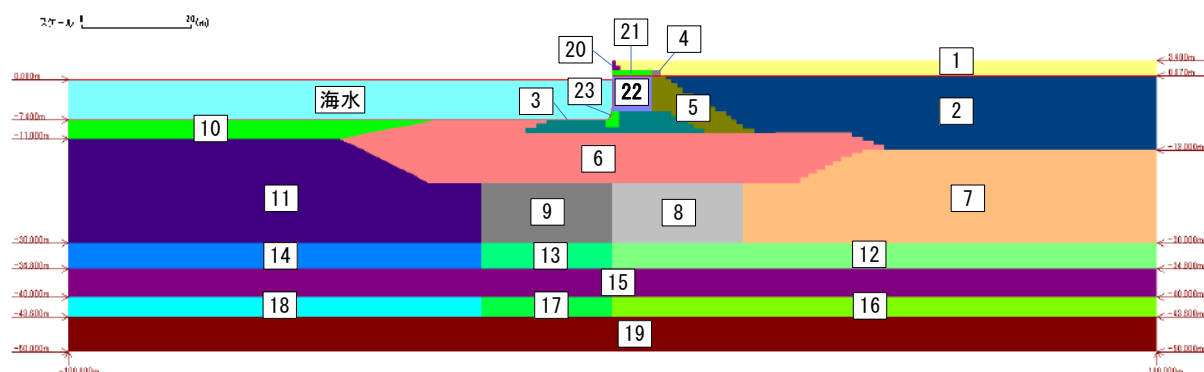
参考図-9.13 土層分割図
