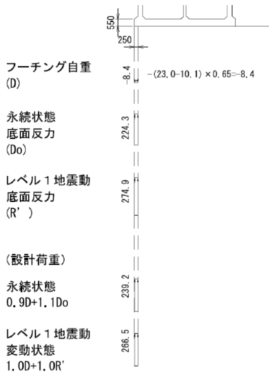
参考図-9.24 フーチングの設計荷重
