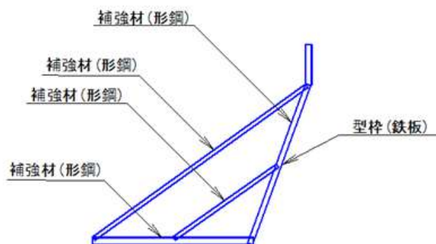
図-5.6.2 鋼製型枠例
