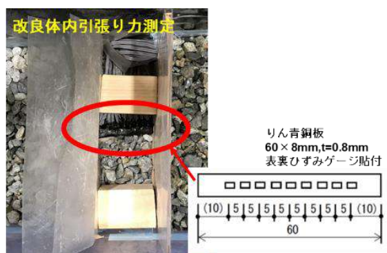
参考写真-6.2 りん青銅板の設置状況
