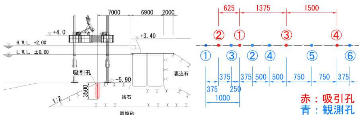
a) 実験位置断面図
